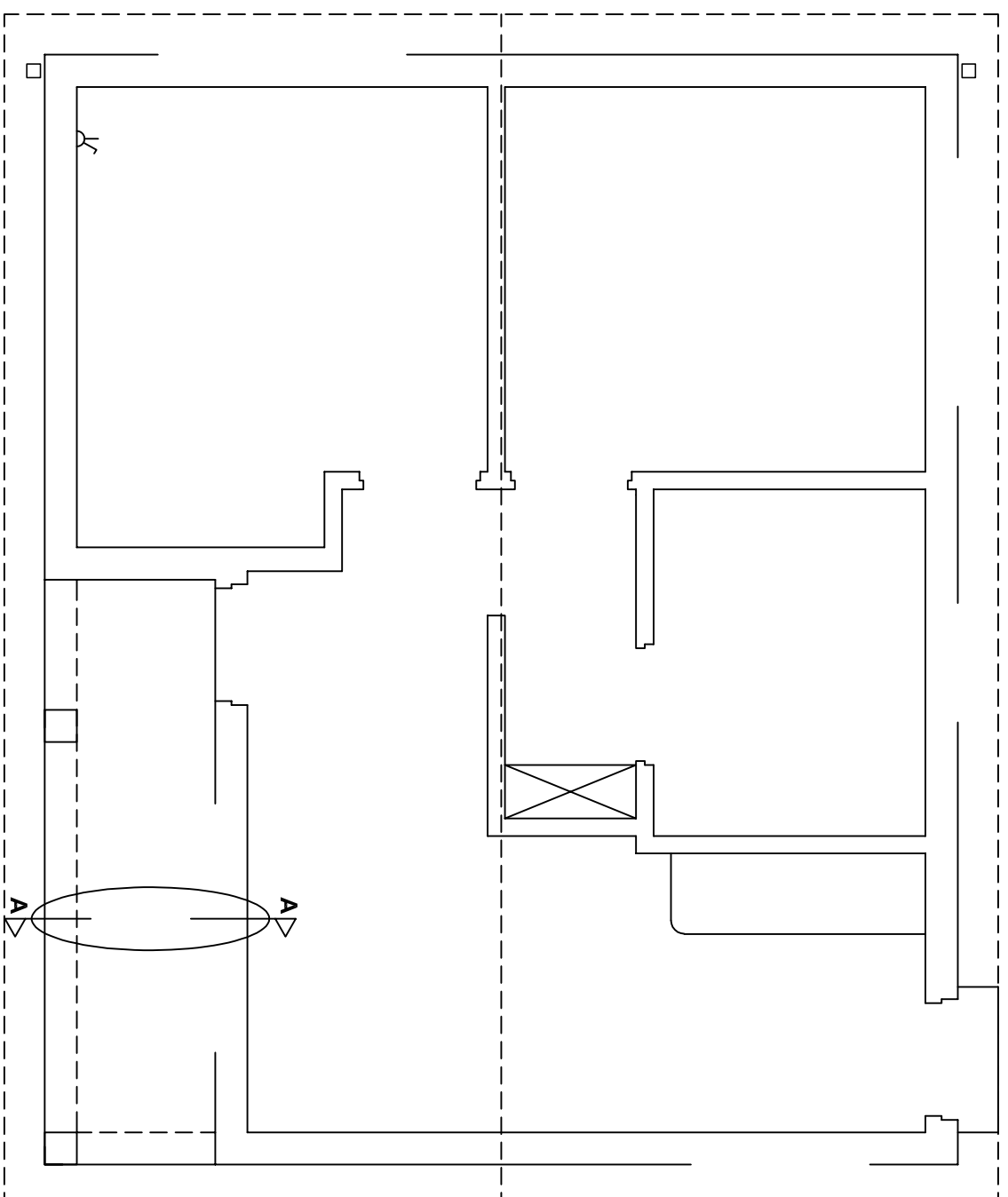
VLOERPLAN SKAAL 1 : 50
